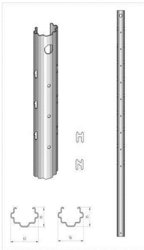
Промежуточные опоры
