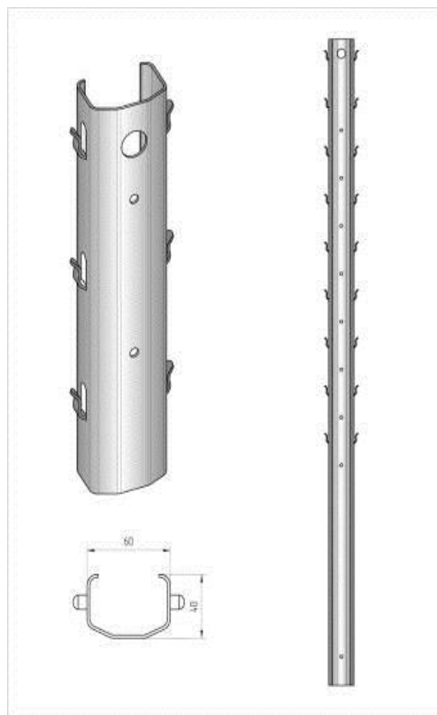
Концевая опора
